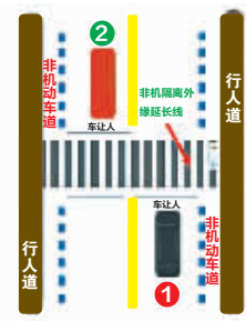
说明 当行人未跨越图中非机动车隔离外缘延长线,1车道上的机动车应停车让行,2车道允许通行。当行人跨越图中非机动车隔离外缘延长线,1和2车道上的机动车应停车让行。
